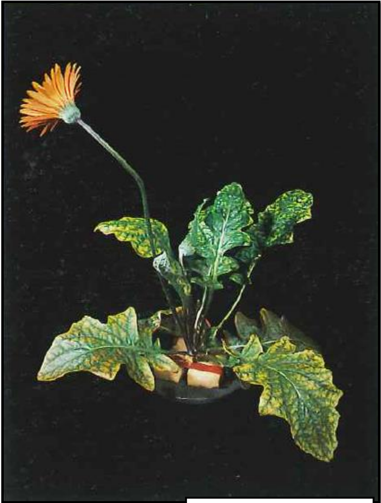
Boriumovermaat (B)
