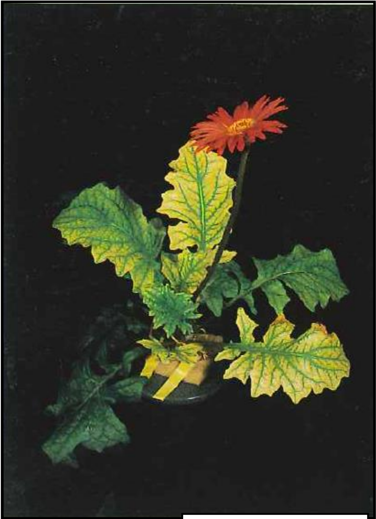
Ijzergebrek (Fe)
