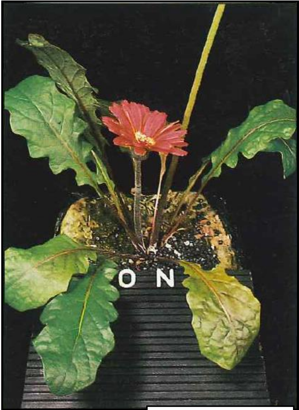
Stikstofgebrek (N)
